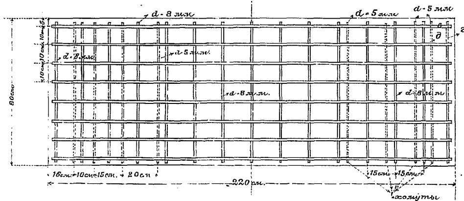
Схема расположения арматуры въ планѣ.
